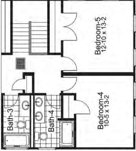
Opt. Bedroom-5 Plan
